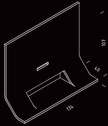
LIR.A wall unit dim. w134 x d40 x h107 cm
