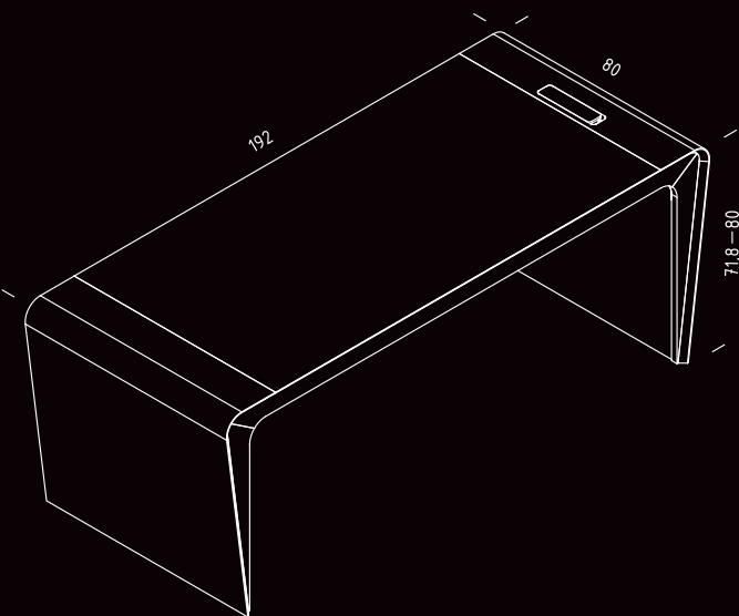
LIR.S desk dim. w192 x d80 x h71,8-80 cm
